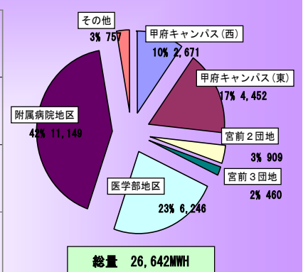
平成21年度電力使用量(MWH)
