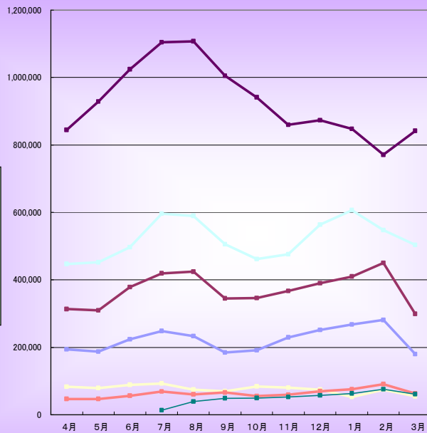
平成21年度電力使用量の月別推移(KWH)
