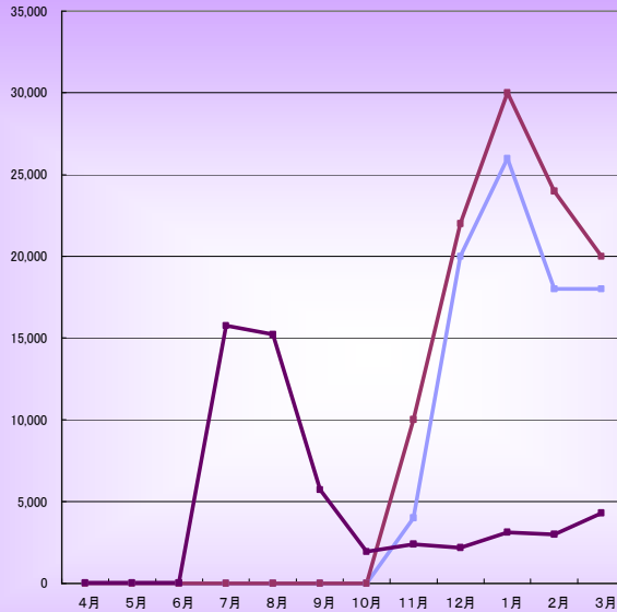
平成21年度重油使用量の月別推移(L)
