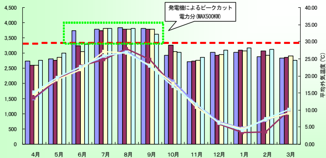
医学部キャンパス 最大電力(KW)
